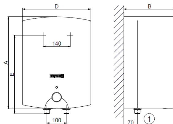
Исполнение над точкой отбора
