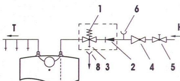
Prevedenie pod odberné miesto
