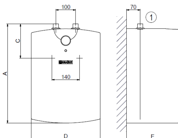
Исполнение под точкой отбора
