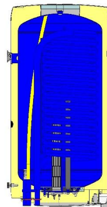
Řez kombinovaným zásobníkem OKHE 125 NTR/DV
