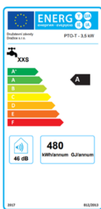
Obr. 2: Energetický štítek se zátěžovým (vytáčecím) profilem
